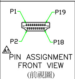
HDMIAC-P4SN (IP66)
