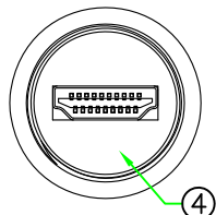
HDMIAC-P4SN (IP66)
