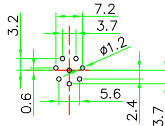
CBD-P108CPF
