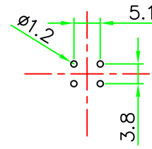
CBD-P104CPF
