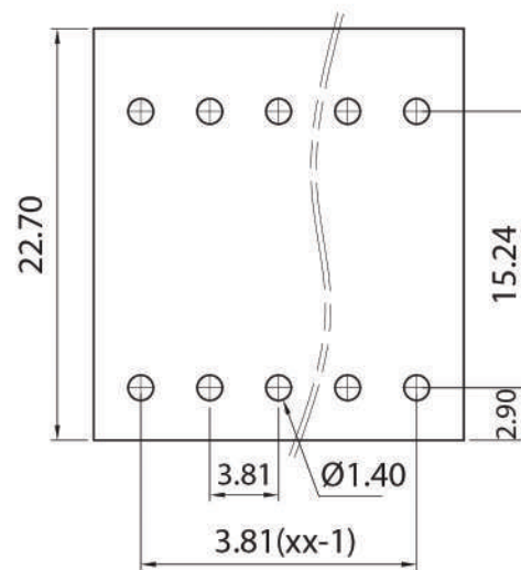
p.c.b. layout
